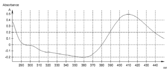
Рисунок 1. Спектр поглощения комплекса рутина с алюминия хлоридом
