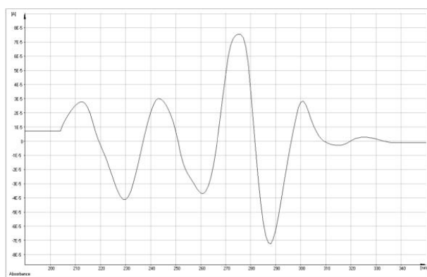
Рисунок 1. Четвёртая производная спектра поглощения дибазола
