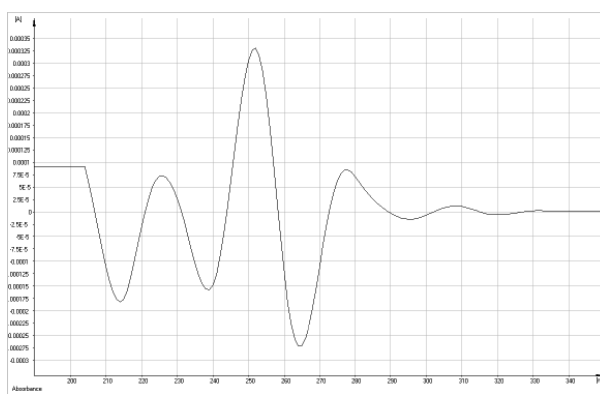
Рисунок 2. Четвёртая производная спектра поглощения папаверина г/х
