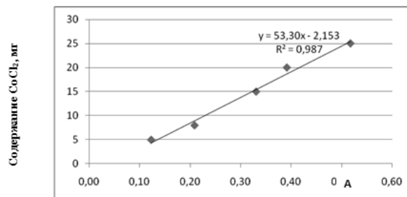
Рисунок 1. Калибровочный график и уравнение пересчета оптической плотности растворов в содержание кобальта хлорида в мг
