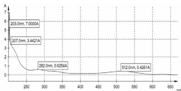
Рисунок 1. Спектр экстракта таблетки с красителями: «Изабелла» и «Черная смородина»
