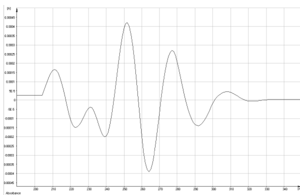
Рисунок 4. Четвёртая производная спектра поглощения смеси веществ
