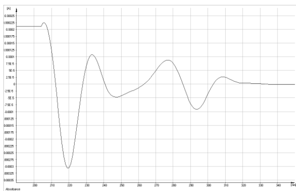
Рисунок 3. Четвёртая производная спектра поглощения теofilлина
