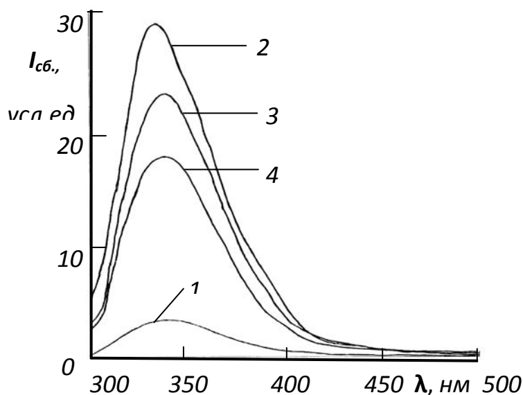
1 – контрольная группа; 2 – реактивная стадия перитонита; 3 – токсическая стадия перитонита; 4 – стадия полиорганной недостаточности Рисунок 1. Характерные спектры флуоресценции сыворотки крови больных перитонитом и контрольной группы I_{сб.} (возбуждение светом с длиной волны 286 нм)
