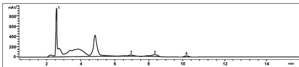
1 – кафтаровая кислота; 2 – робинин; 3 – пара-кумаровая кислота; 4 – цикориевая кислота Рисунок 2 – Хроматограмма спиртового извлечения из корней эхинацеи пурпурной, заготовленной на территории Республики Беларусь
