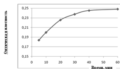
Рисунок 2. Зависимость оптической плотности растворов комплекса алюминия хлорида с рутином от времени
