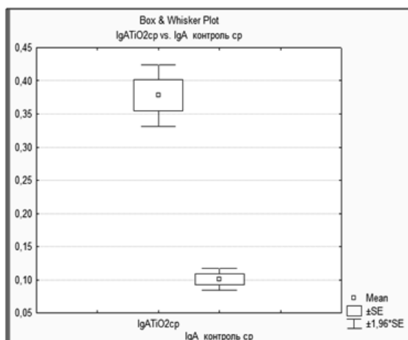
Рисунок 1. Достоверность различий по доверительным интервалам между оптической плотностью лунок с TiO_2 и контролем (луночки тест-системы без красителя)
