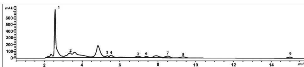
1 – кафтаровая кислота; 2 – хлорогеновая кислота; 3 – кофейная кислота; 4 – рутин; 5 – робинин; 6 – хирзутрин; 7 – пара-кумаровая кислота; 8 – синаповая кислота; 9 – орто-кумаровая кислота Рисунок 1 Хроматограмма спиртового извлечения из травы эхинацеи пурпурной, заготовленной на территории Республики Беларусь
