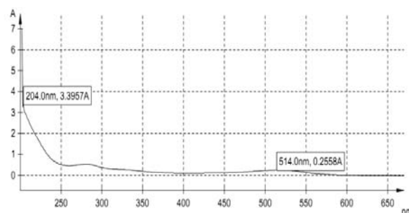
Рисунок 2. Спектр экстракта таблетки без красителей
